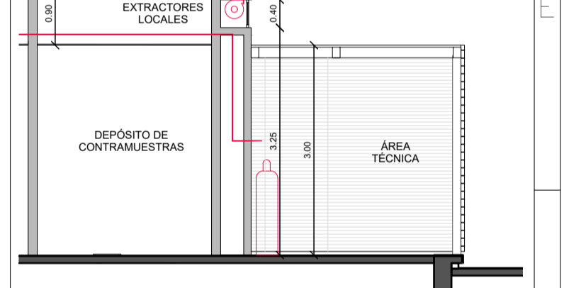
CORTE POR NICHOS EXTRACTORES LOCALES
